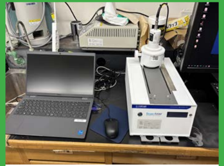
Scan-RAM TLC スキャナー (LabLogic Systems 社)
